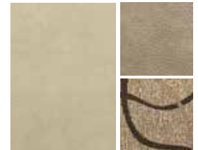
VANILLA
